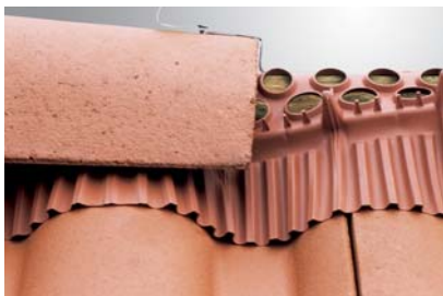
Automatische Formgebung durch Aufsetzen des Firststeines.
